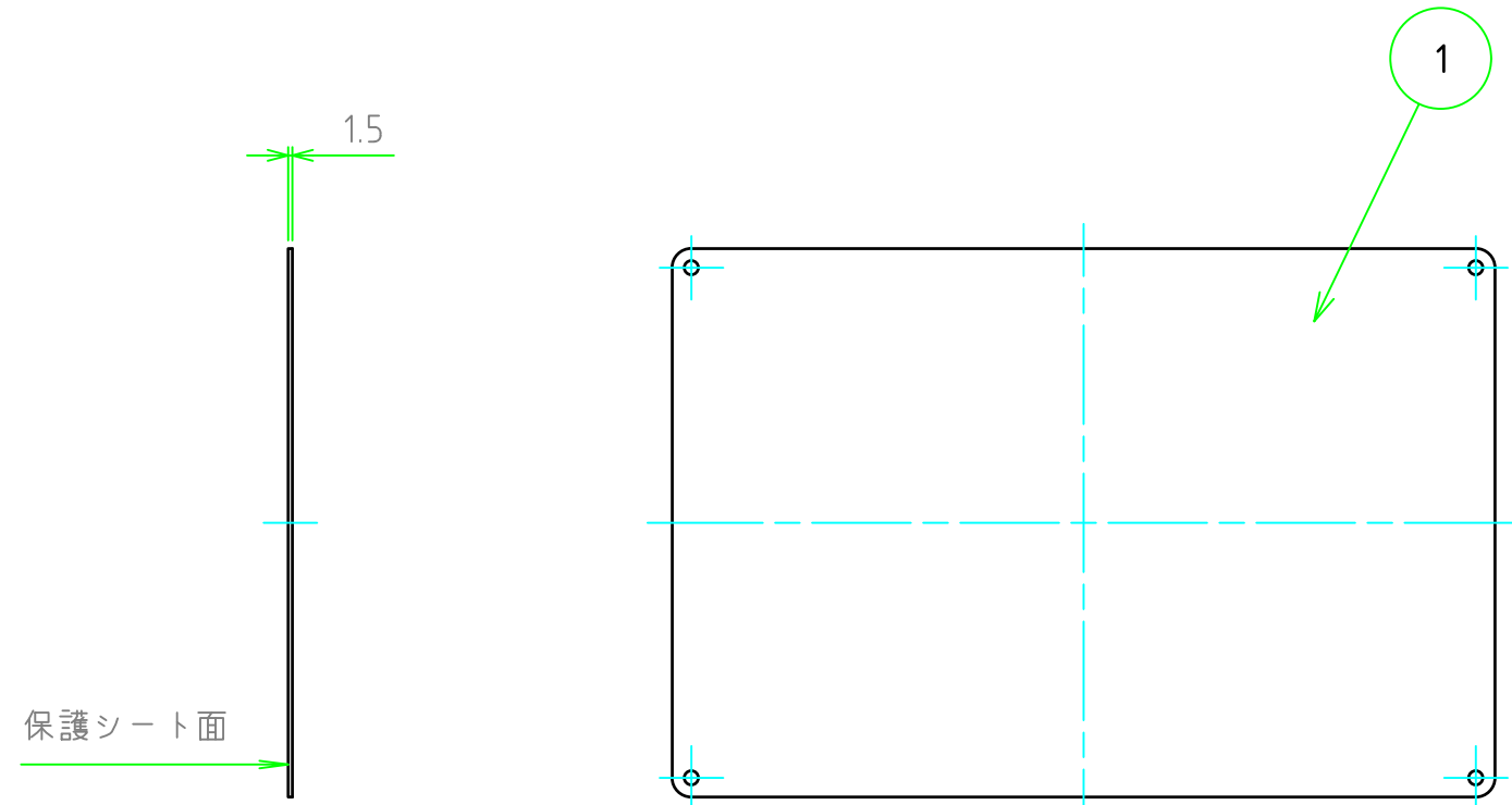
パネル裏面
