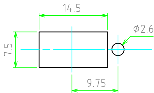
取付穴寸法
