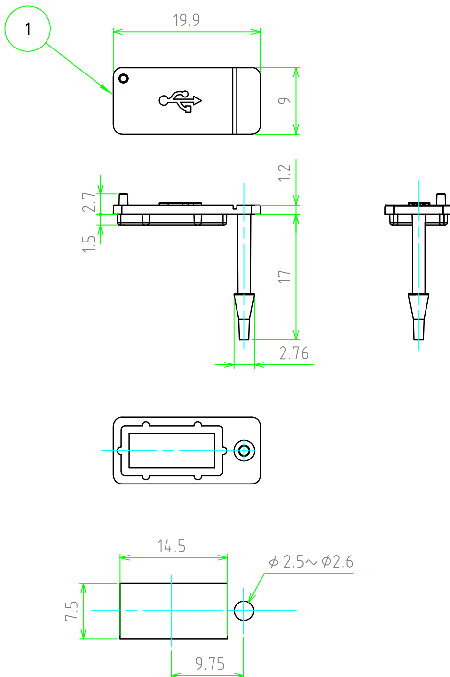
取付穴寸法
