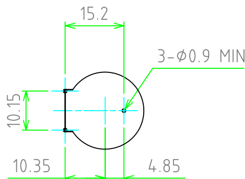
基板取付穴ピッチ PCB layout top view
