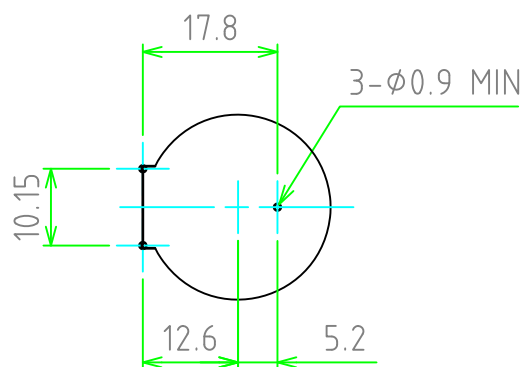
基板取付穴ピッチ PCB layout top view
