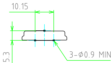
基板取付穴ピッチ PCB layout top view
