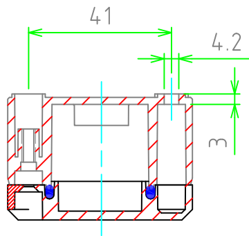
C-C（外部取付穴詳細図）
