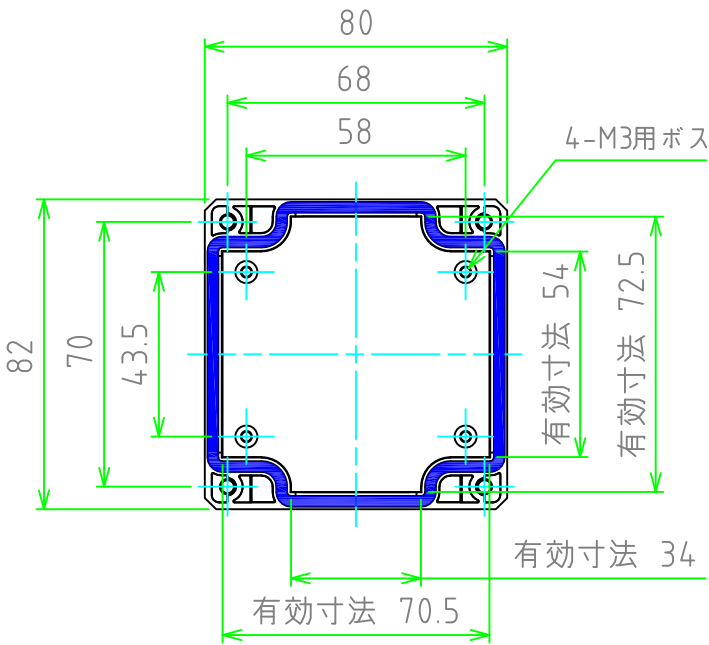
カバー（内視）
