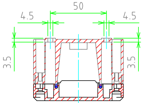
C-C（外部取付穴詳細図）
