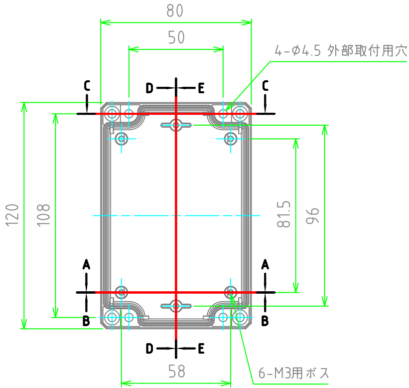
ボディー(内視)
