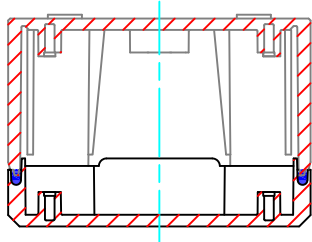
A-A
