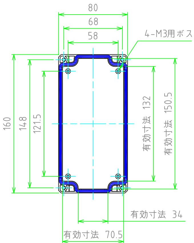
カバー（内視）
