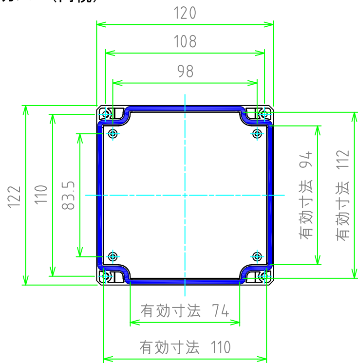
カバー（内視）
