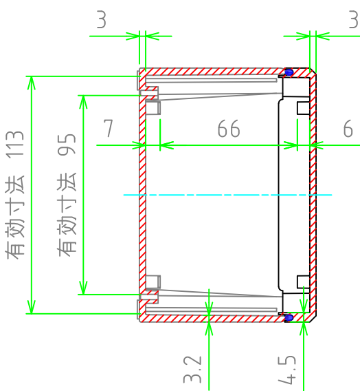
D-D
