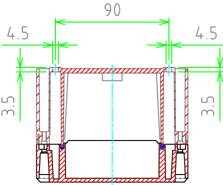
C-C (外部取付穴詳細図)
