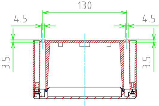
C-C (外部取付穴詳細図)
