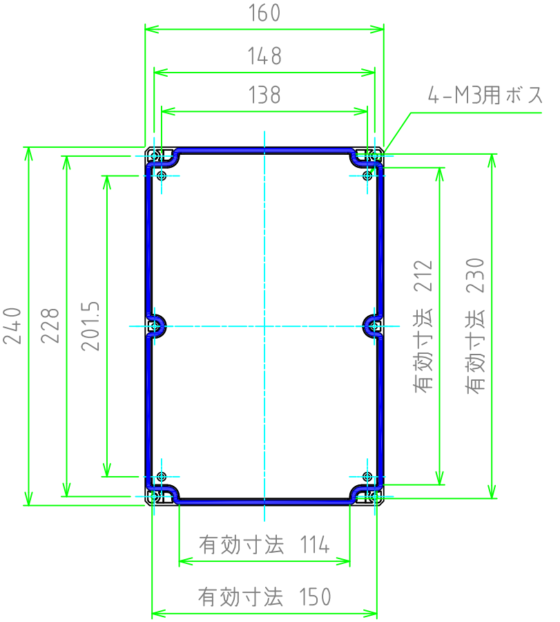
カバー(内視)
