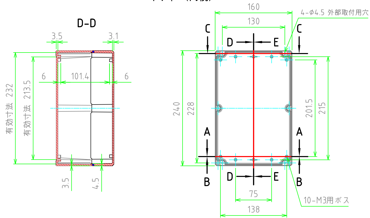
ボディ（内視）
