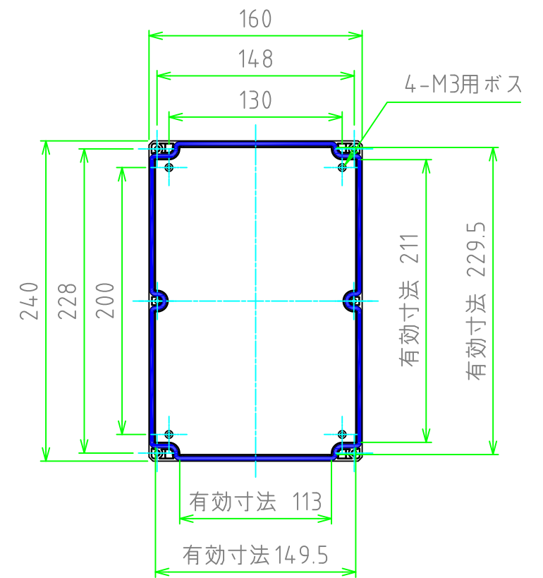
カバー（内視）
