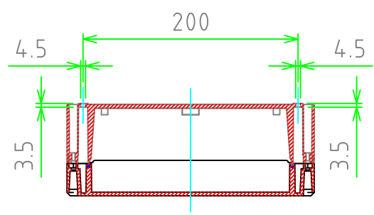
C-C（外部取付穴詳細図）
