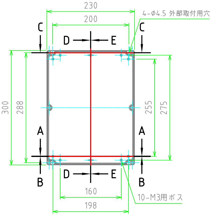
ボディ(内視)
