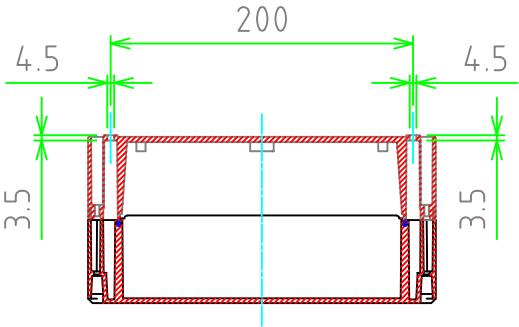
C-C (外部取付穴詳細図)
