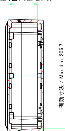
A-A (1:3)
