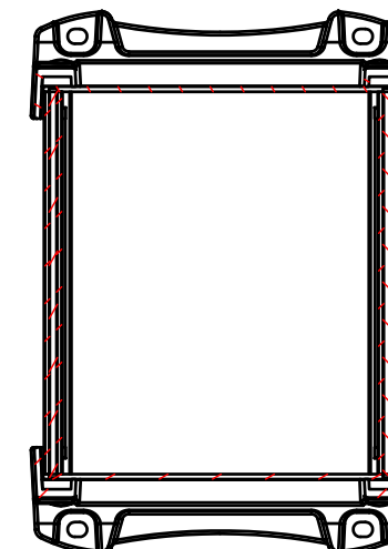
D-D (1:2.5)
