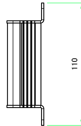
C-C (1:2)
