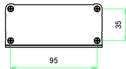
A-A ( 1 : 2.5 )
