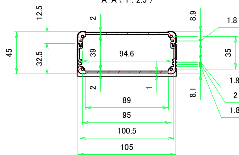
A-A ( 1 : 2.5 )
