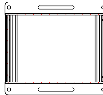
C-C ( 1 : 2.5 )
