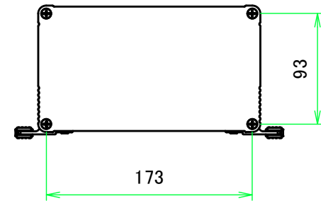
A-A ( 1 : 4.5 )
