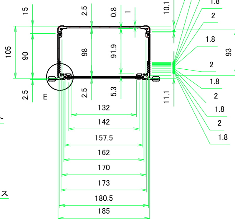
A-A ( 1 : 4.5 )
