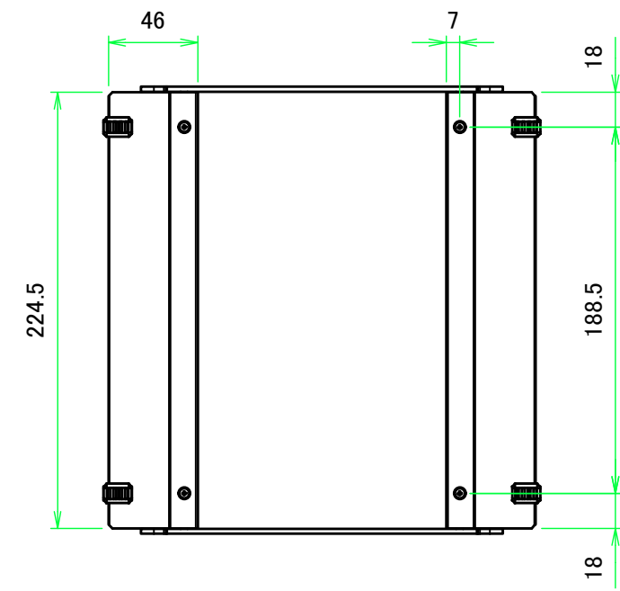
D-D (1:3.5)
