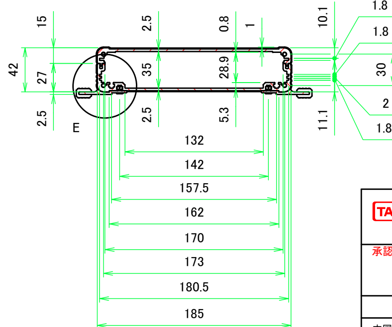
A-A (1:3.5)
