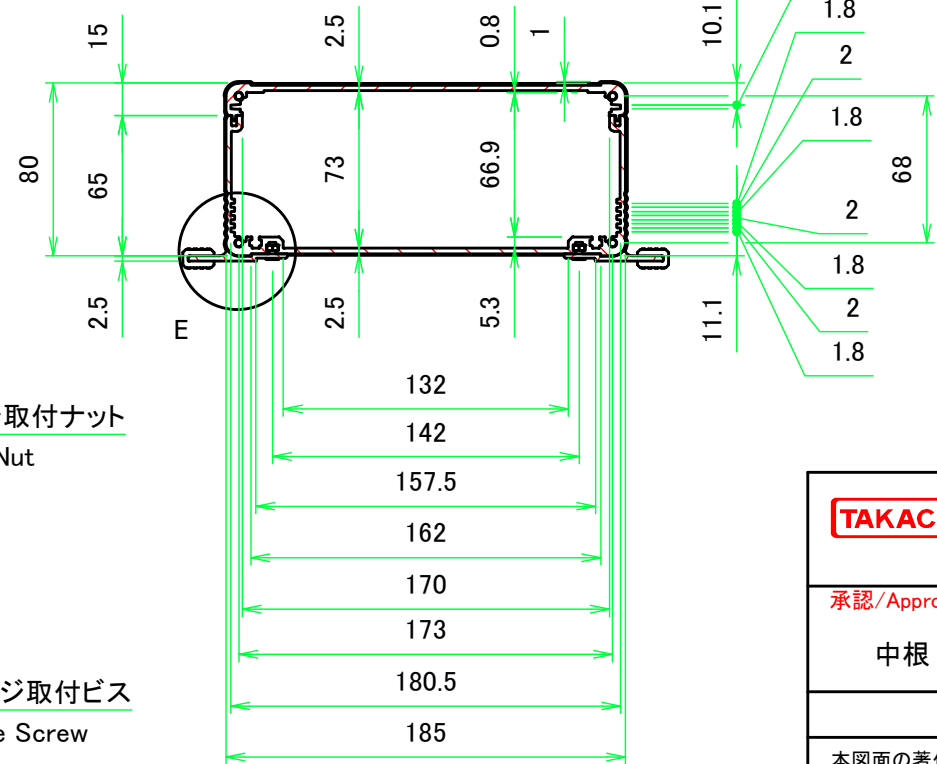
A-A (1:3.5)
