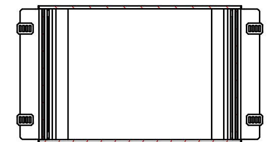
D-D (1:3.5)
