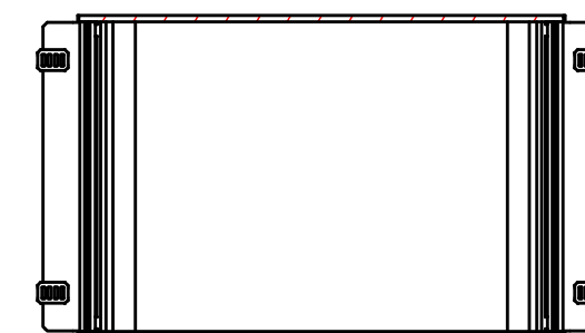
D-D (1:4)
