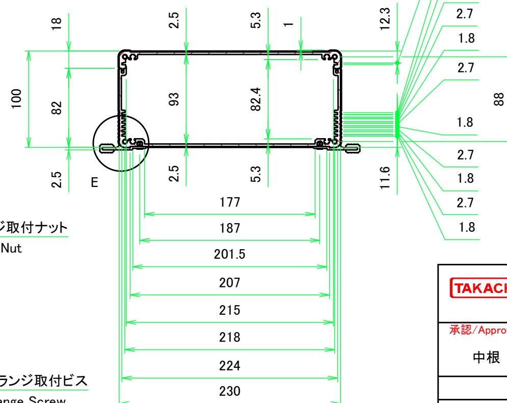
A-A (1:4)
