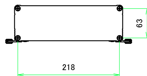
A-A (1:5)
