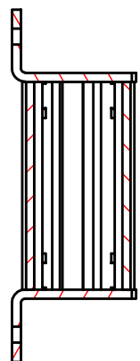
B-B ( 1 : 1.5 )
