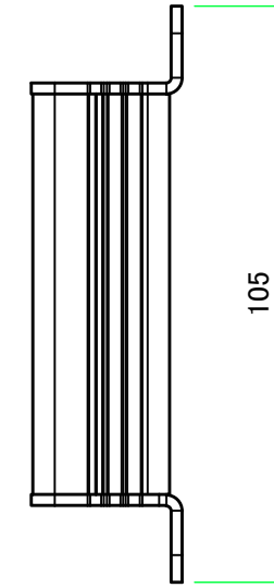
C-C ( 1 : 1.5 )
