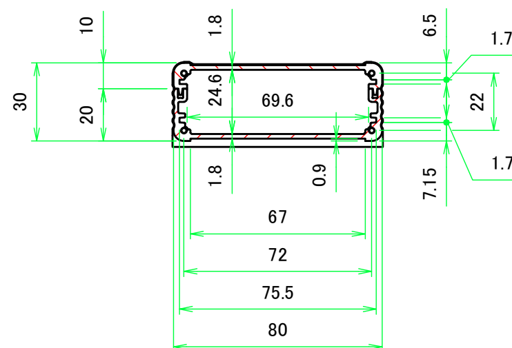
A-A (1:2)
