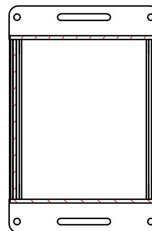
C-C (1:2)
