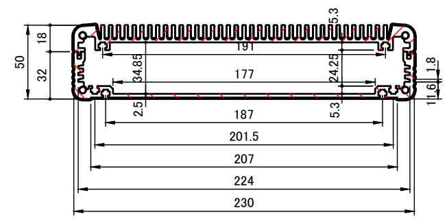
A-A (1:3.5)
