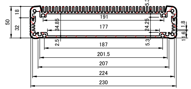
A-A (1:3.5)
