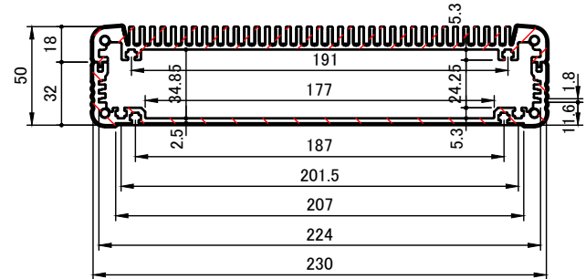
A-A (1:3.5)
