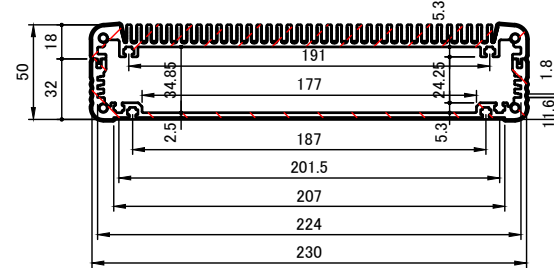
A-A (1:4)
