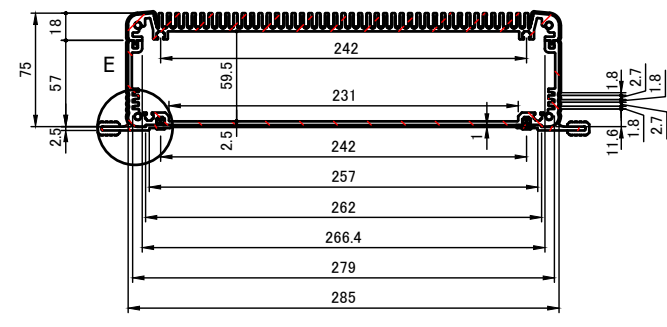
A-A (1:5)
