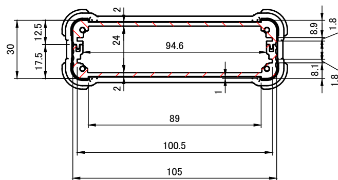
A-A (1:2)
