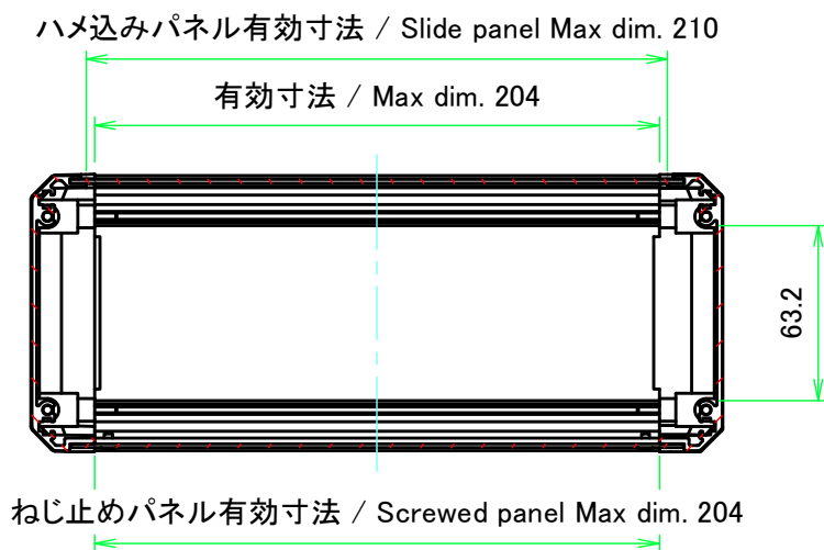
A-A (1:3)
