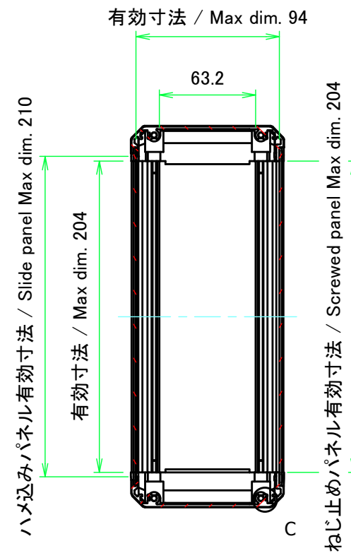
B-B (1:3.5)
