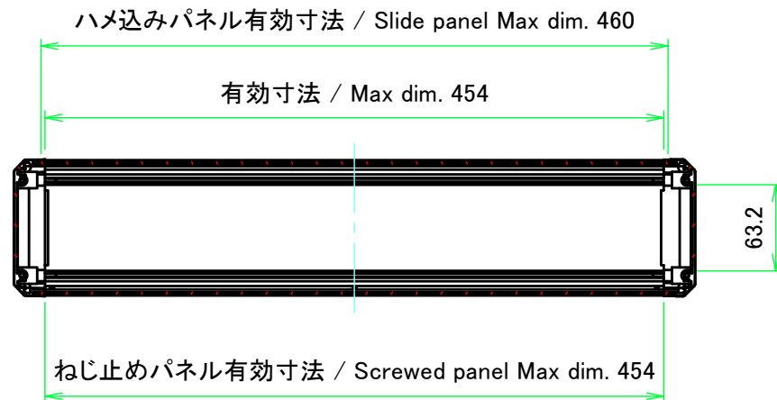
A-A (1:5)
