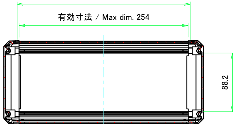
A-A (1:3.5)
