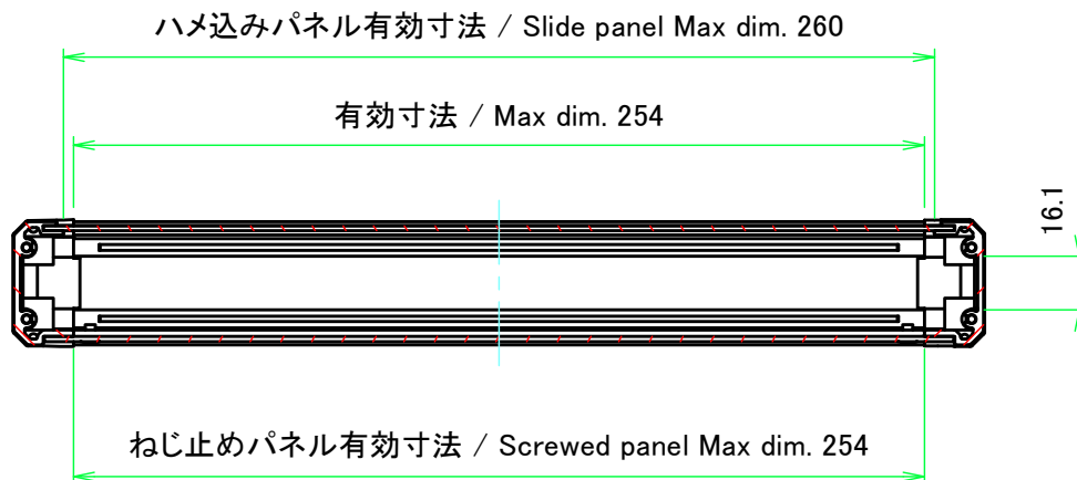
A-A (1:2.5)
