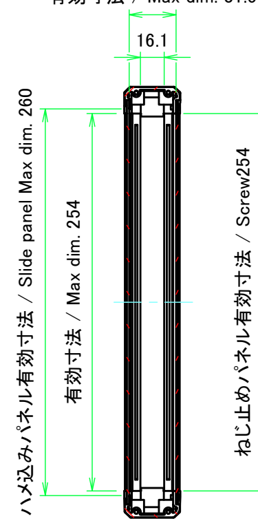
B-B (1:3.5)
