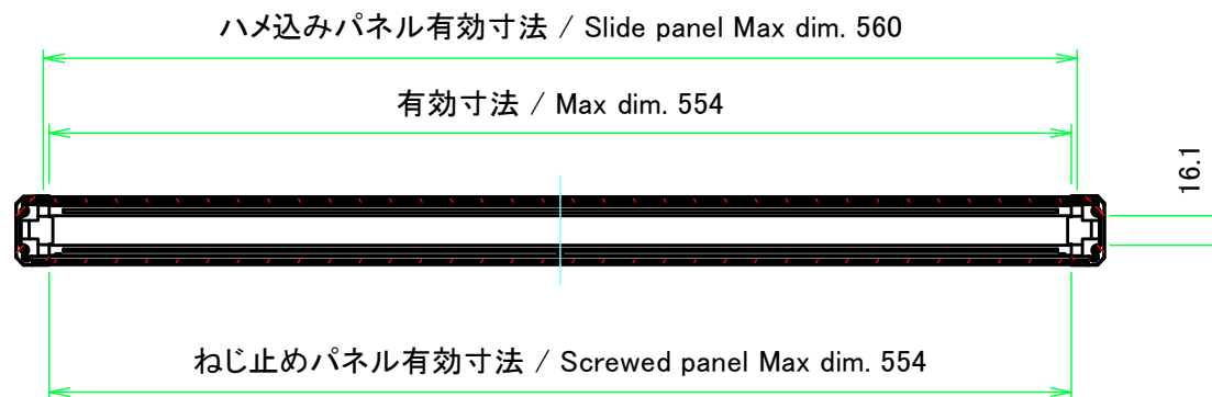
A-A (1:4.5)
