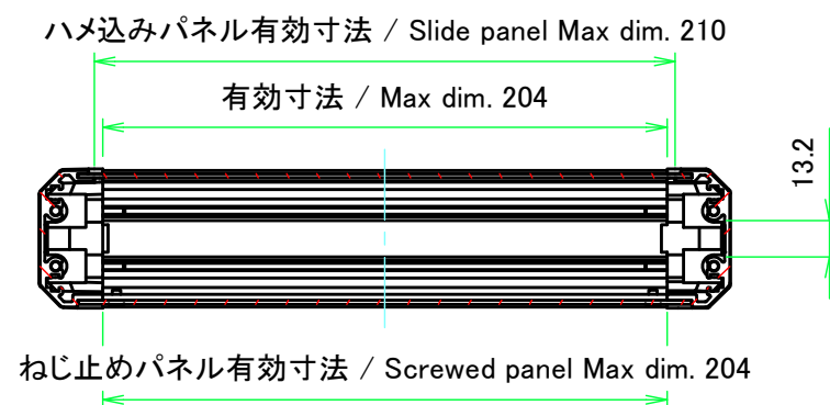
A-A (1:3)
