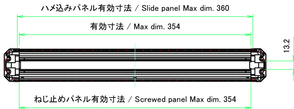
A-A (1:3.5)
