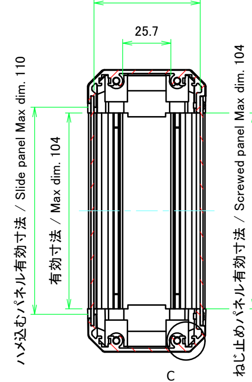
B-B (1:2)
