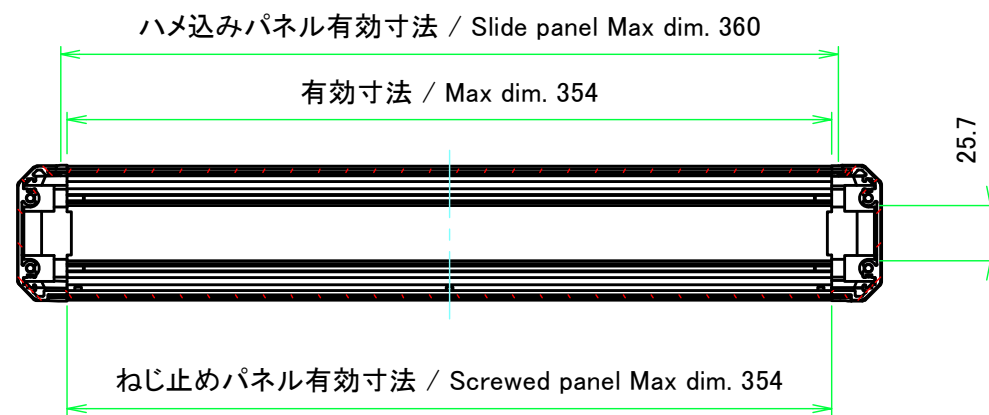
A-A (1:3.5)
