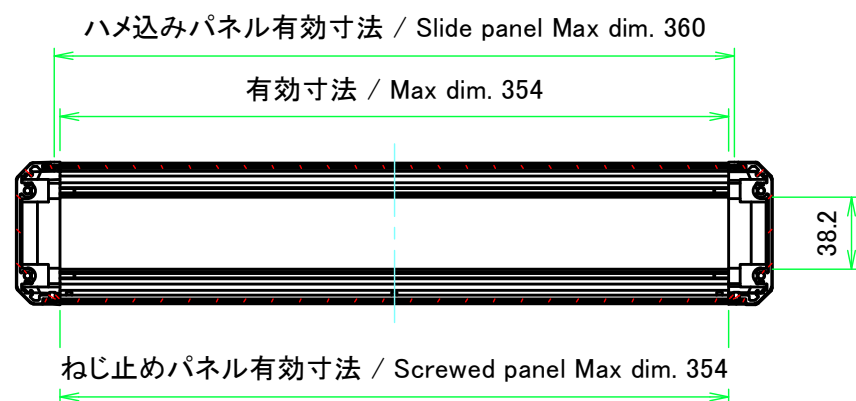
A-A (1:4)
