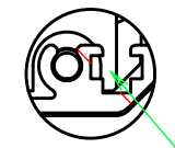
C : フレーム拡大図 / Frame cross-section
