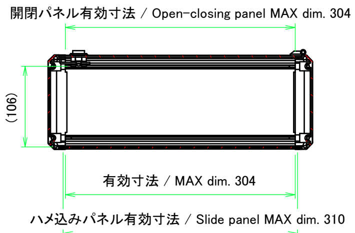
A-A (1:5)
