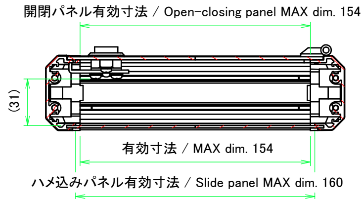
A-A (1:2.5)
